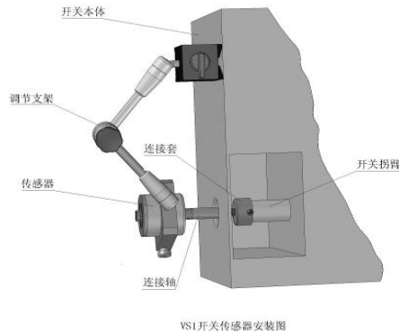
VS1 开关传感器安装图
